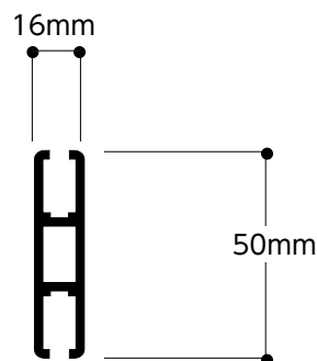
ビーム断面図
